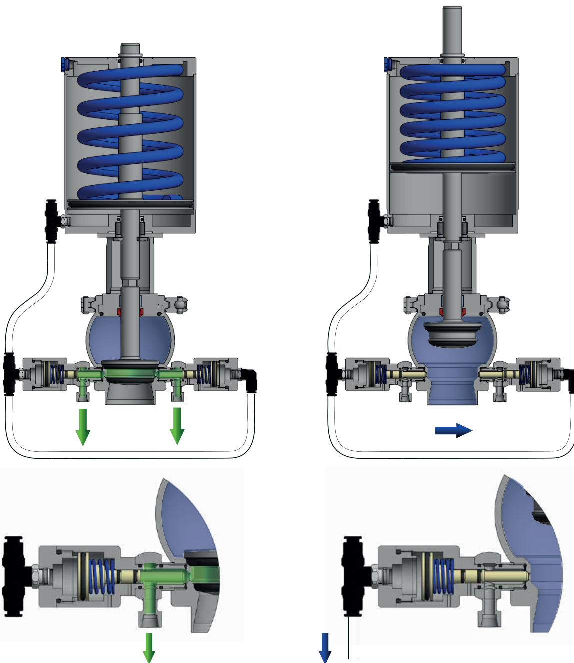
Fig. 1 VALVOLA CHIUSA
