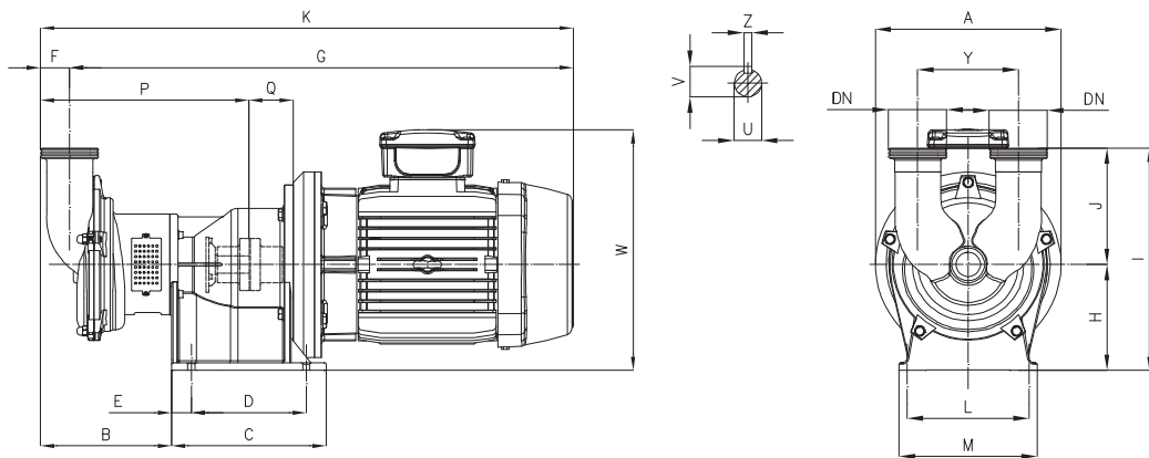
Mesures non contractuelles - DN = Raccords femelle DIN 11851 - Exécution avec moteur standard IEC - EN (* Support préparé pour accouplement moteur ...)
