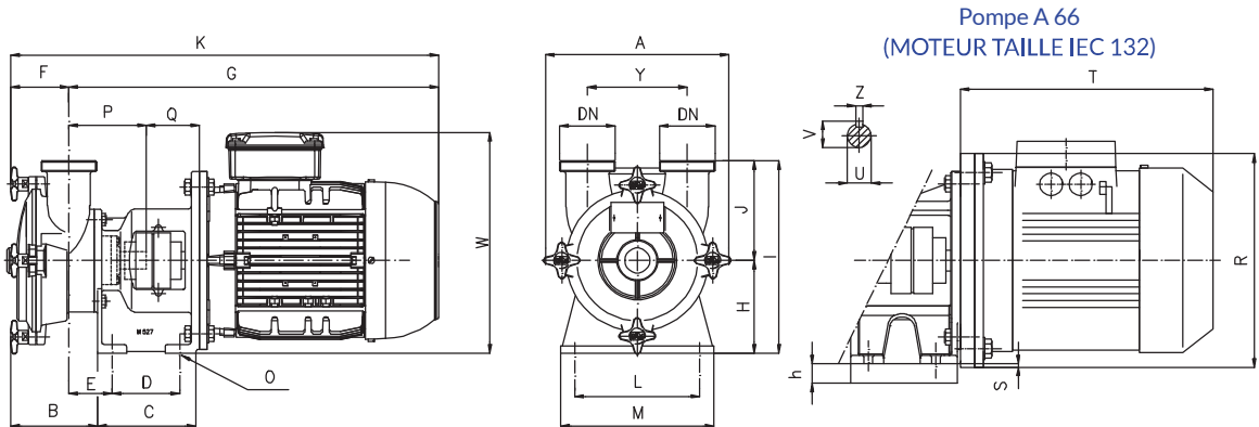
Mesures non contractuelles - DN = Raccords femelle DIN 11851 - Exécution avec moteur standard IEC - EN (* Support préparé pour accouplement moteur ...)
