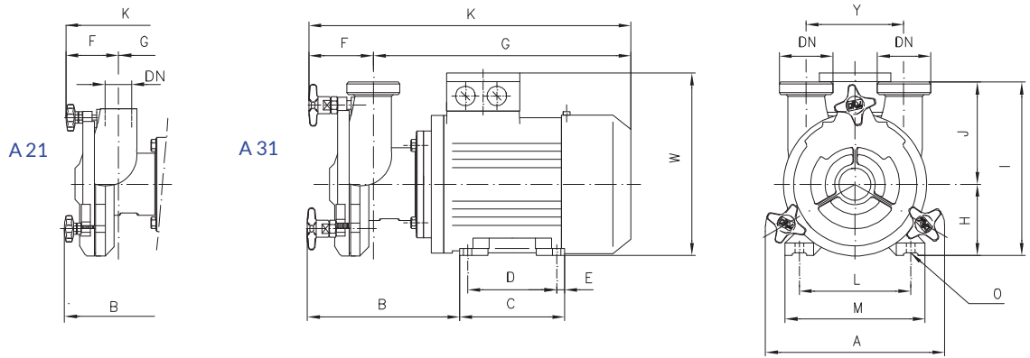
Mesures non contractuelles - DN = Raccords GAZ pour A 21 Raccords femelle DIN 11851 pour A 31
